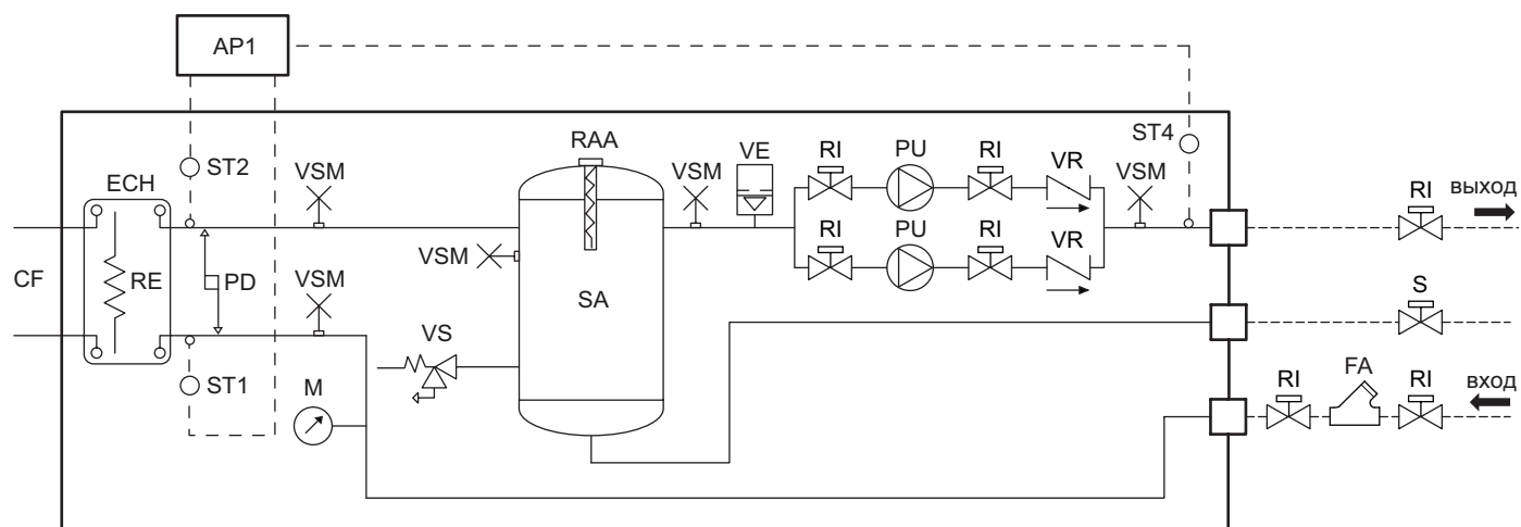
TCAEY-THAEY 245÷265 ASDP1 – ASDP2
