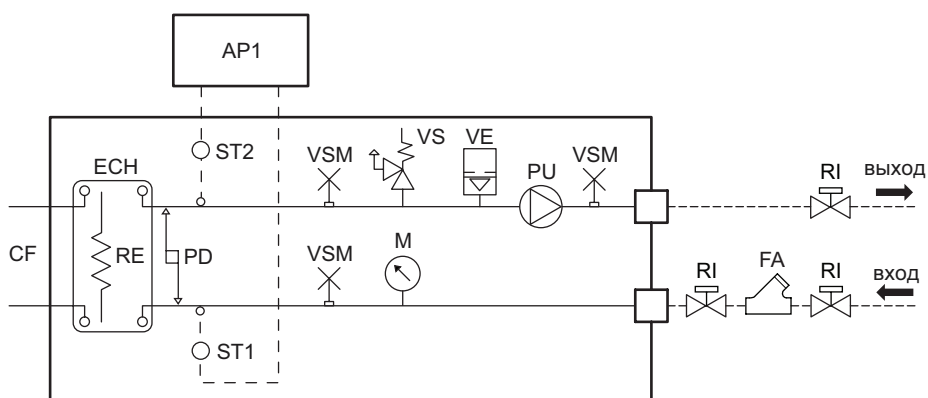
ТСАЕУ-ТНАЕУ 245÷265 P1 – P2
