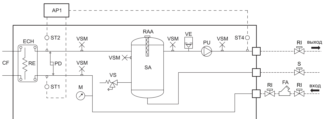
ТСАЕУ-ТНАЕУ 245÷265 ASP1 – ASP2
